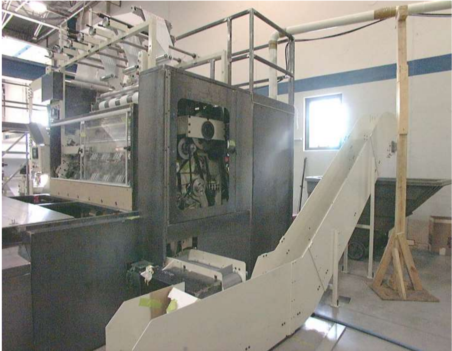
072-Folder
